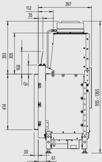
Zijaanzicht
