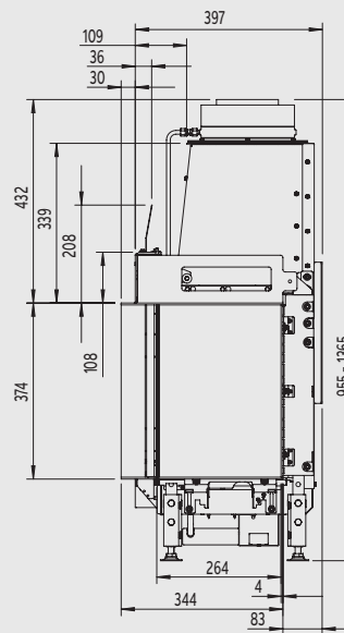
Zijaanzicht
