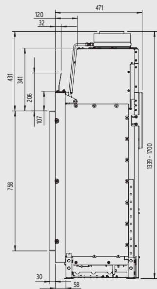
Zijaanzicht
