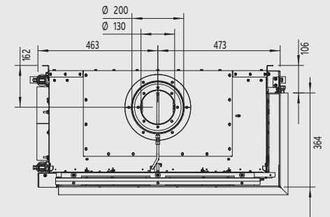
Zijaanzicht
