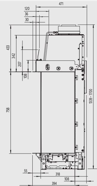
Zijaanzicht
