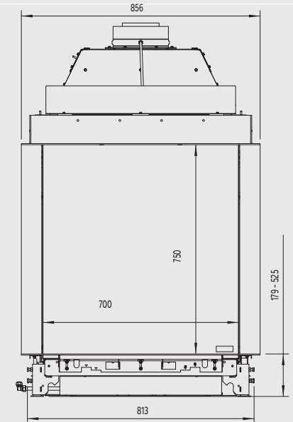
Bovenzijde
