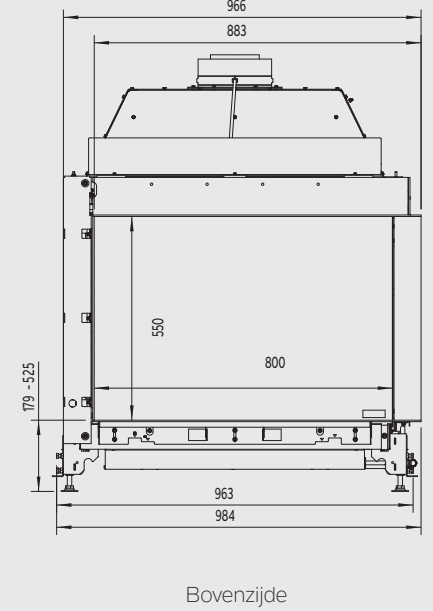
Voorzijde
