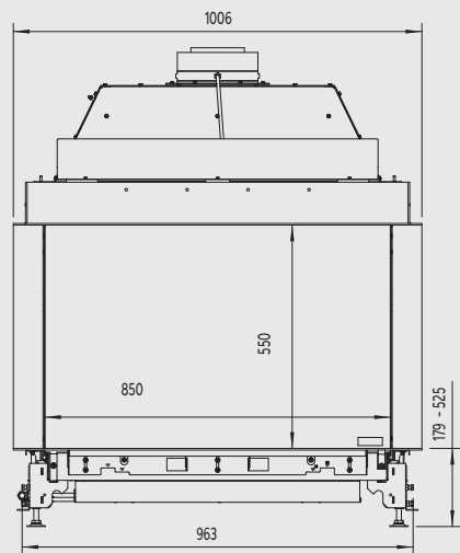
Bovenzijde
