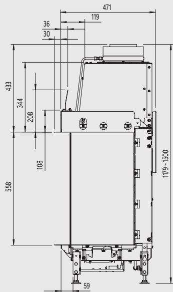
Zijaanzicht
