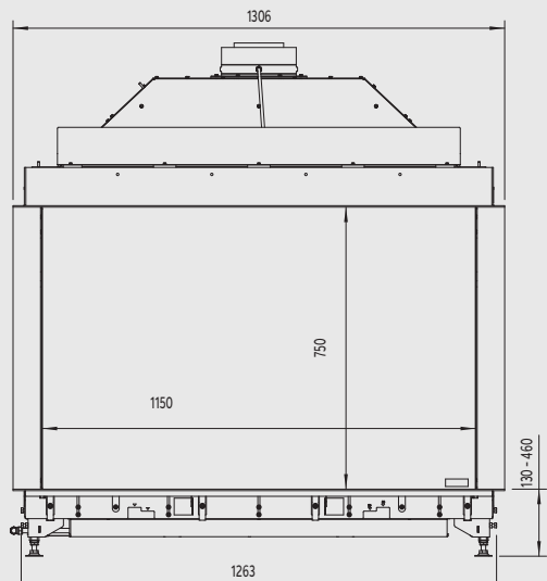
Bovenzijde
