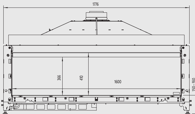
Bovenzijde
