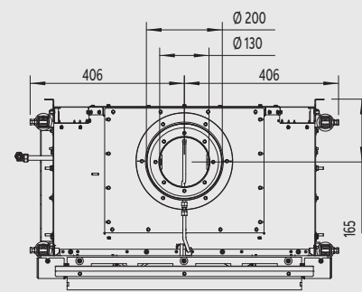
Zijaanzicht
