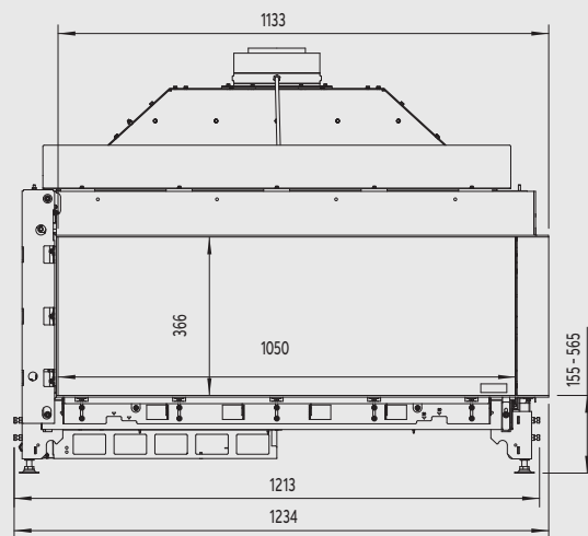
Bovenzijde
