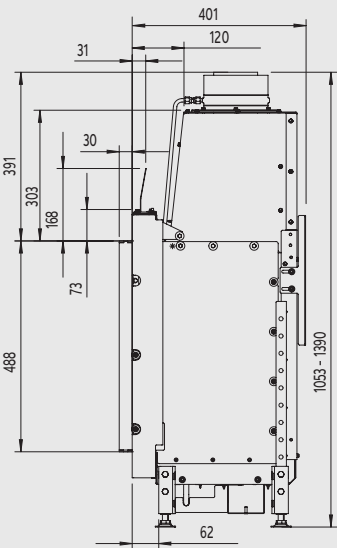
Zijaanzicht
