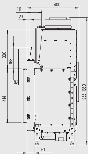
Zijaanzicht
