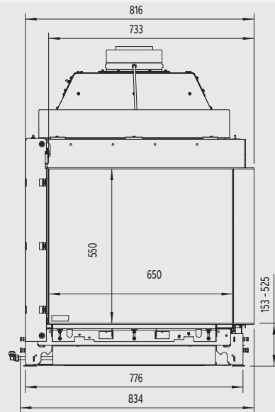
Bovenzijde
