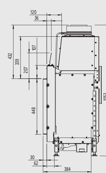
Zijaanzicht
