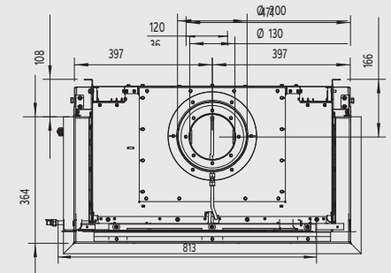
Zijaanzicht
