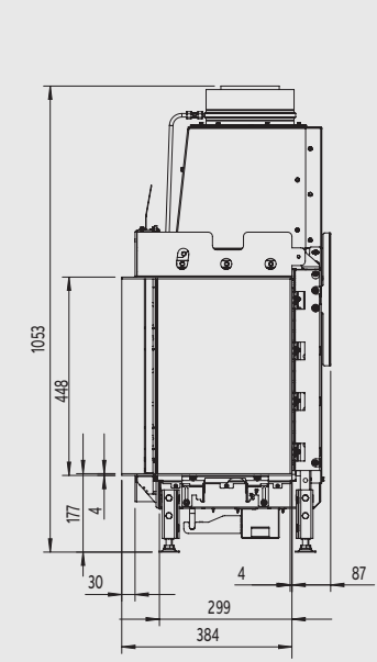
Zijaanzicht
