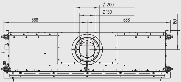
Zijaanzicht
