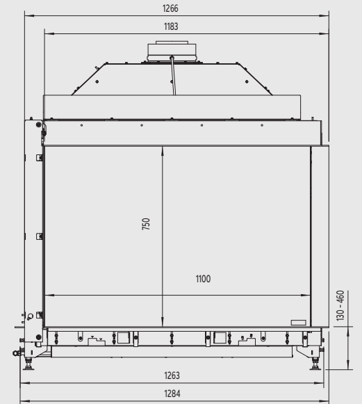
Bovenzijde
