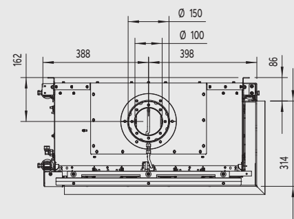
Zijaanzicht
