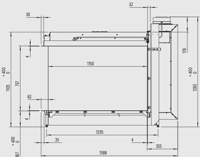
Bovenzijde
