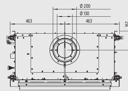
Zijaanzicht
