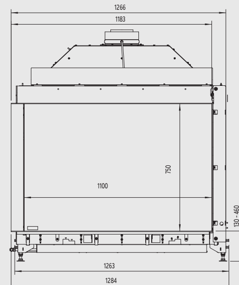
Bovenzijde
