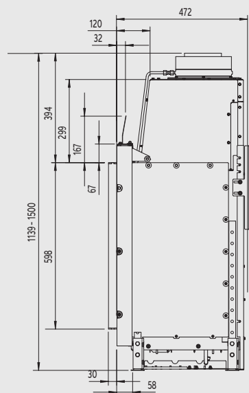
Zijaanzicht
