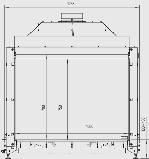
Bovenzijde
