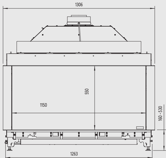
Bovenzijde
