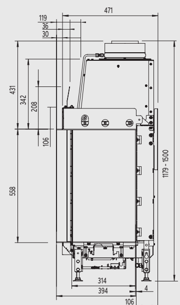
Zijaanzicht
