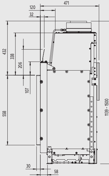
Zijaanzicht
