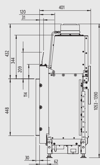
Zijaanzicht
