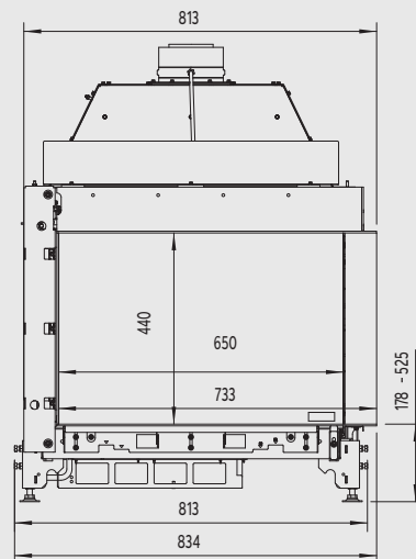
Bovenzijde
