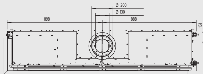
Zijaanzicht
