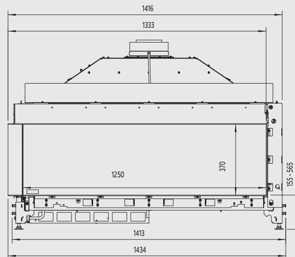
Bovenzijde
