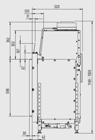
Zijaanzicht
