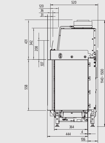
Zijaanzicht
