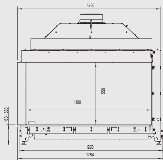
Bovenzijde
