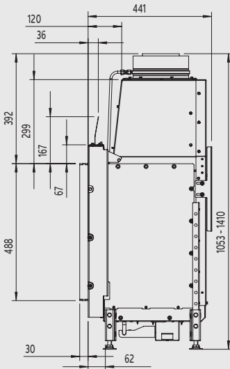
Zijaanzicht
