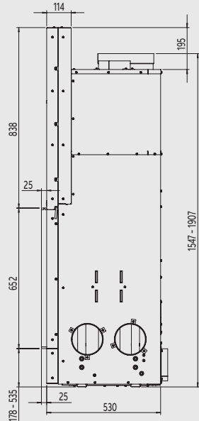
Zijaanzicht
