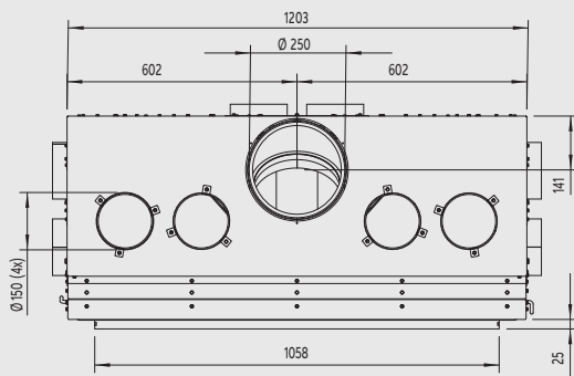
Zijaanzicht
