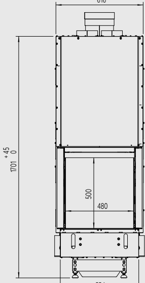
Bovenzijde
