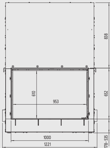
Bovenzijde
