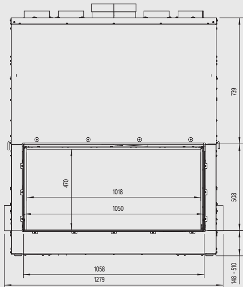
Bovenzijde
