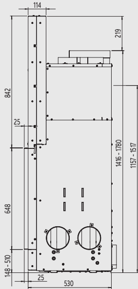
Zijaanzicht
