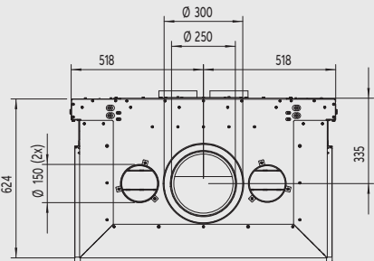
Zijaanzicht
