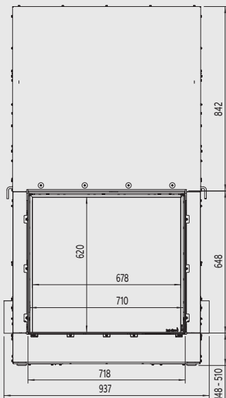
Bovenzijde
