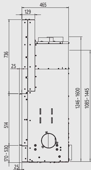
Zijaanzicht
