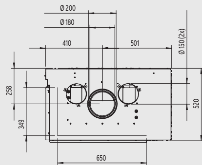
Zijaanzicht
