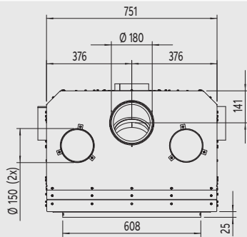
Zijaanzicht
