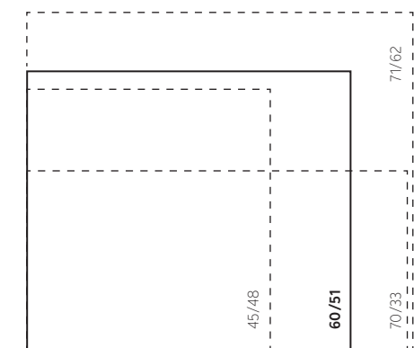
Glasmaten fronthaarden
