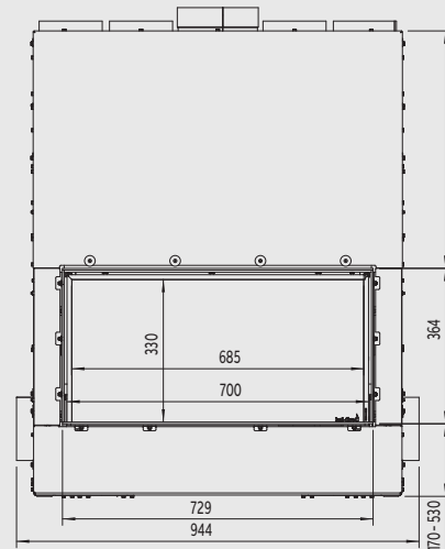
Bovenzijde
