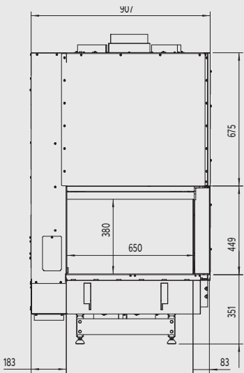
Bovenzijde
