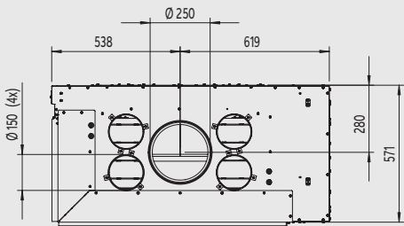
Zijaanzicht
