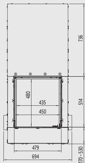
Bovenzijde
