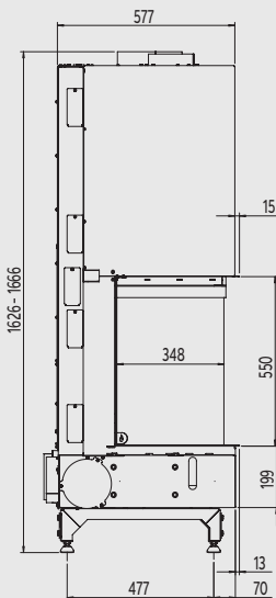
Zijaanzicht
