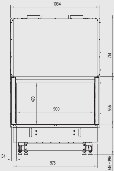
Bovenzijde
