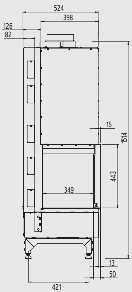
Zijaanzicht
