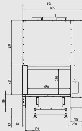
Bovenzijde
