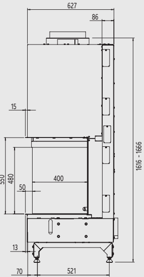
Zijaanzicht
