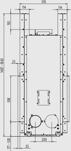
Zijaanzicht
