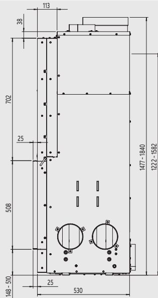
Zijaanzicht
