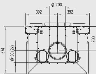
Bovenzijde
