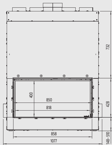
Bovenzijde
