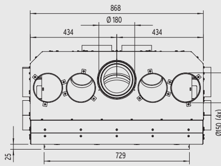
Zijaanzicht
