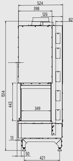
Zijaanzicht
